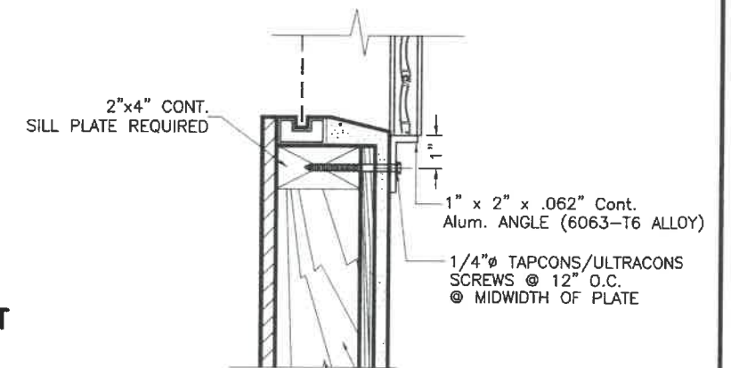
SECTION X-X SCALE: 3/8" = 1"
